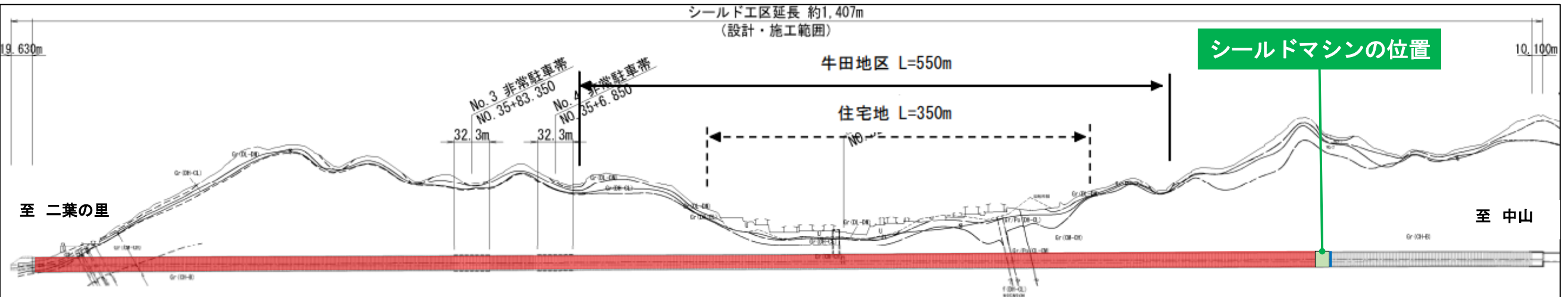
縦断図
